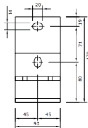
Vooraanzicht muursteun wandmontage
