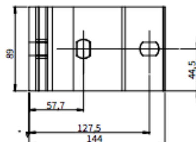
Bovenaanzicht plafondsteun
